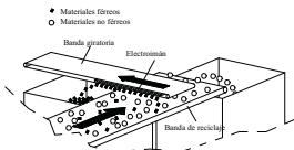
Dibujo 17: Principio de funcionamiento del electroimán
