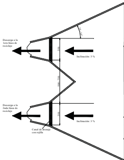
Dibujo 13: Tolva recibidora grande
