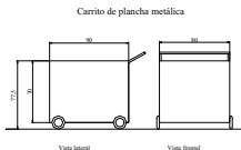
Dibujo 19: Carritos manuales
