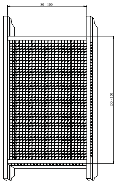
Dibujo 2: Tamiz para análisis de basura
