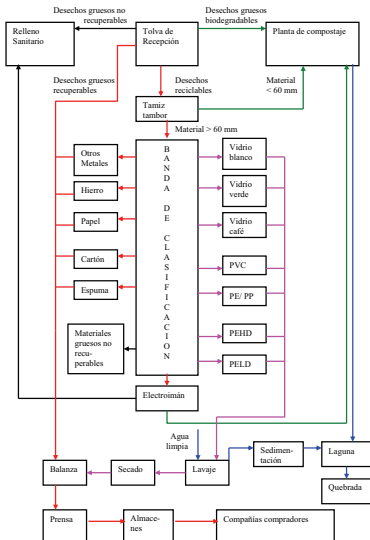
Dibujo 9: Diagrama de Flujo Planta de reciclaje mecanizada
