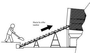
Dibujo 14: Suministro de la criba tambor con una banda giratoria
