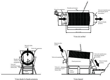
Dibujo 15: Criba Tambor
