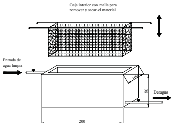
Dibujo 7: Piscina de lavado de plásticos
