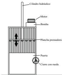
Dibujo 24: Prensa hidráulica
