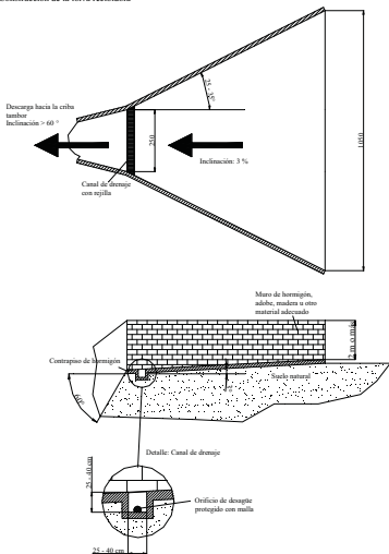
Dibujo 12: Tolva recibidora
