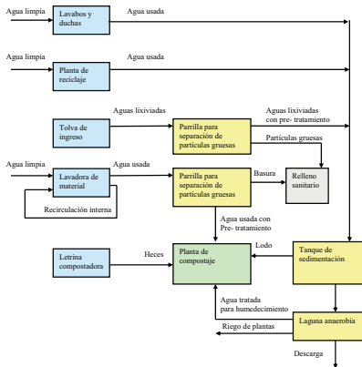
Dibujo 31: Flujo de agua con letrina compostadora
