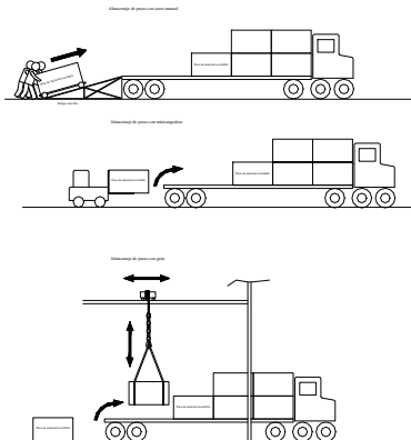
Dibujo 29: Carga de bultos con carro manual, con montacargas y con grúa
